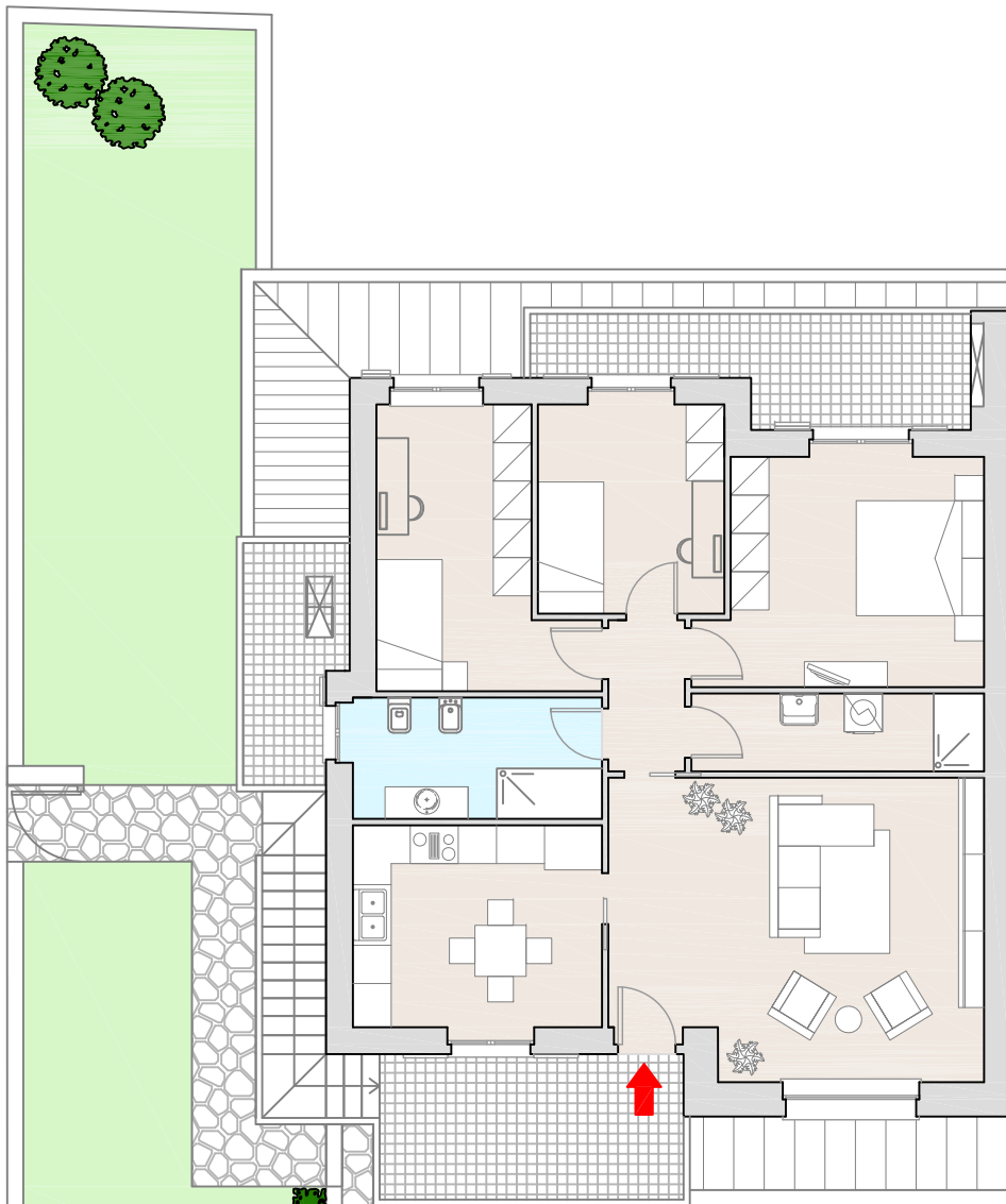
Piano Primo
